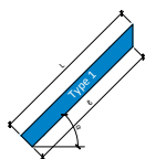
Verticale afschuining nok Toegelaten helling 0° tot 58°
