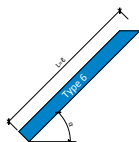
Horizontale afschuining nok Toegelaten helling 32° tot 90°
