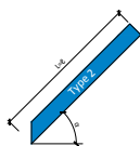
Verticale afschuining goot Toegelaten helling 0° tot 58°
