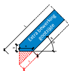
Verticale & horizontale afschuining goot (basisafschuining verticaal => verlenging z) Toegelaten helling 32° tot 58°
